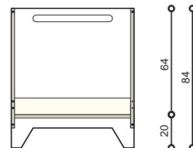
Schnitt Matratze unten
